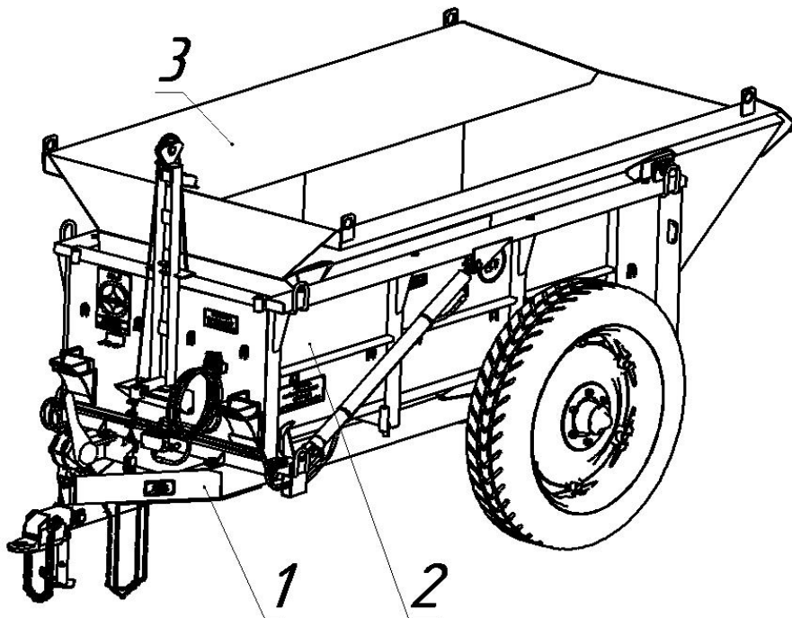
Fig.5. Atașamentul pentru transportarea poamei pe șasiul agregatului modular STMR-18-2000: 1 – modul șasiu; 2 – modul-basculant; 3 – atașament-benă pentru transportarea poamei
