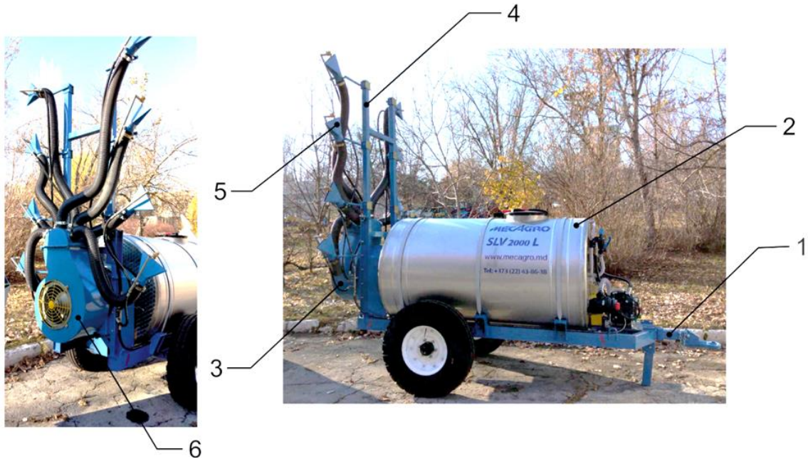
Fig. 3. Mașină de stropit SLV-2000L cu ventilare-pulverizare locală 1 –cadru-șasiu; 2 – rezervor 2m 3 ; 3 – duză de refulare (inferioare); 4 –cadru vertical ; 5 –duze de refulare (superioare); 6 – ventilator centrifugal
