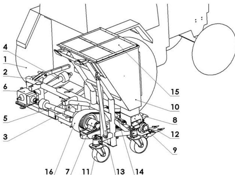
Fig.8.Vederea generală a toculatorului de crengi și coarde de viță-de-vie din grămezi.
