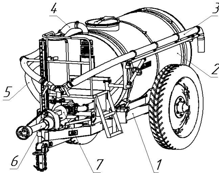
Fig.4. Modulul-agregat pentru transportarea apei, montat în cadrul sistemului STMR-18-2000 1 – modul-șasiu; 2 – rezervor 2\text{m}^3 ; 3 –furtun de livrare; 4 –furtun de umplere a rezervorului; 5 – furtun de absorbție; 6 –arbore cardanic; 7 –pompă
